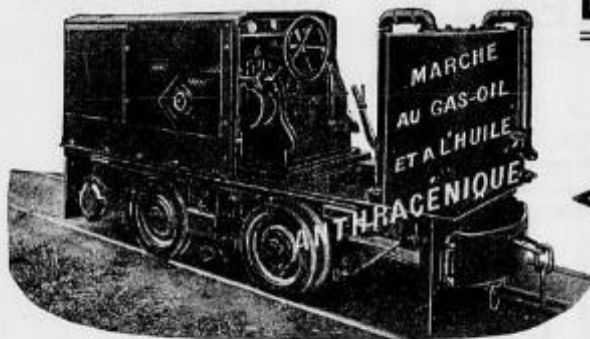
Locomotive Diesel Montania de Mines Type LD7 — 20 CV Agrée pour les mines grisouteuses et poussiéreuses par le Ministère des Travaux Publics
