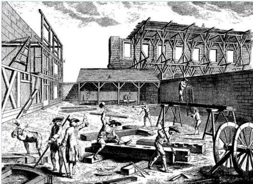
Illustrations : Encyclopédie de Diderot et d'Alembert – Planches Charpente et Architecture
