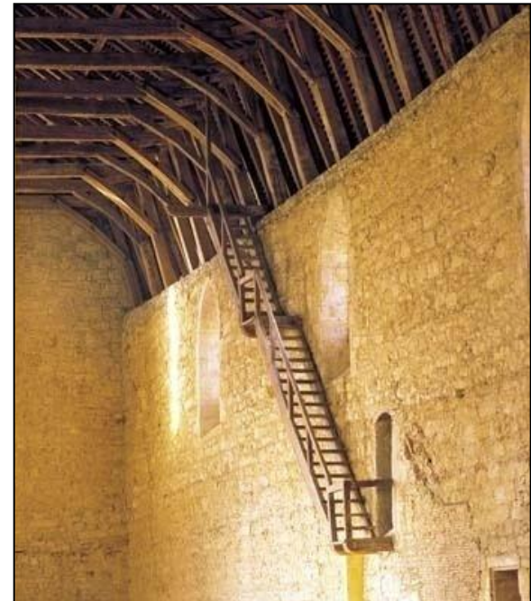
Charpente du couvent des Cordeliers de Saint-Nizier-sous-Charlieu (XVII e siècle). Photo Société des Amis des Arts de Charlieu.
