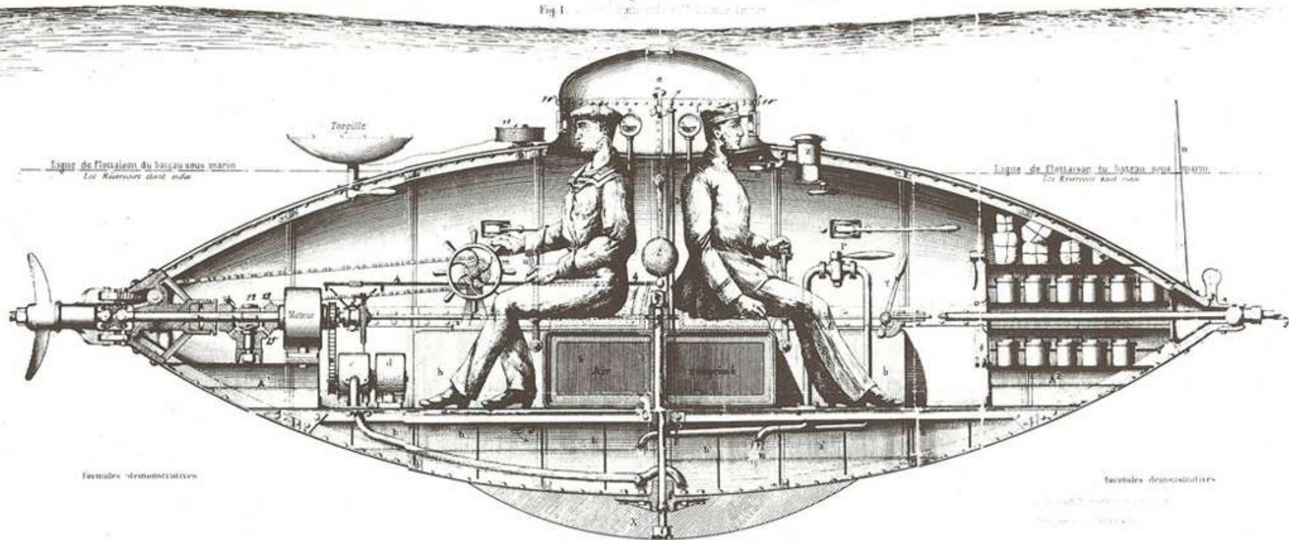
BATEAU TORPILLE R. SOUS-MARIN. Brevet de Propriété C. GOUBET, AIN, le 26 Mars 1885, en France et à l'Étranger. Fig. 1.
